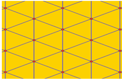
Figura 16. Teselado a partir de triángulos equiláteros.
